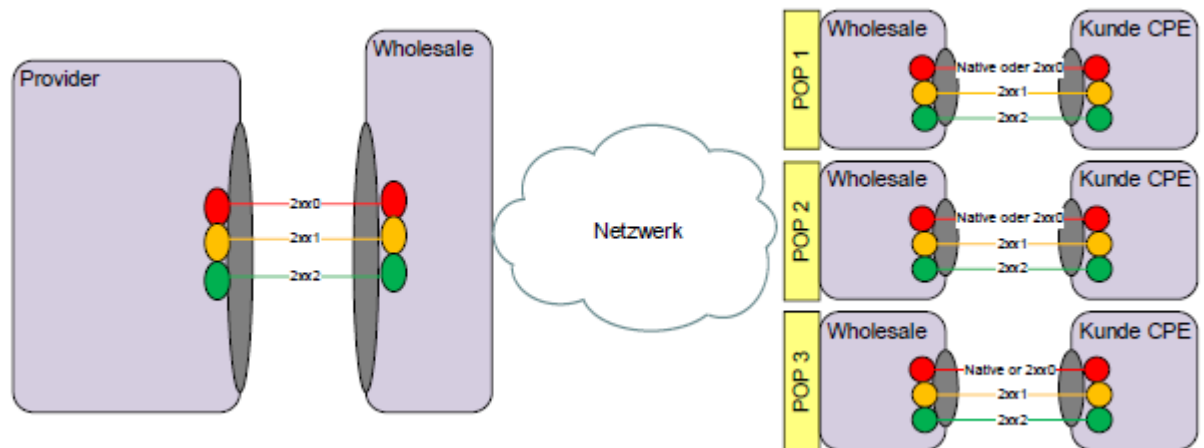
Abbildung 5 VLAN-Konzept
