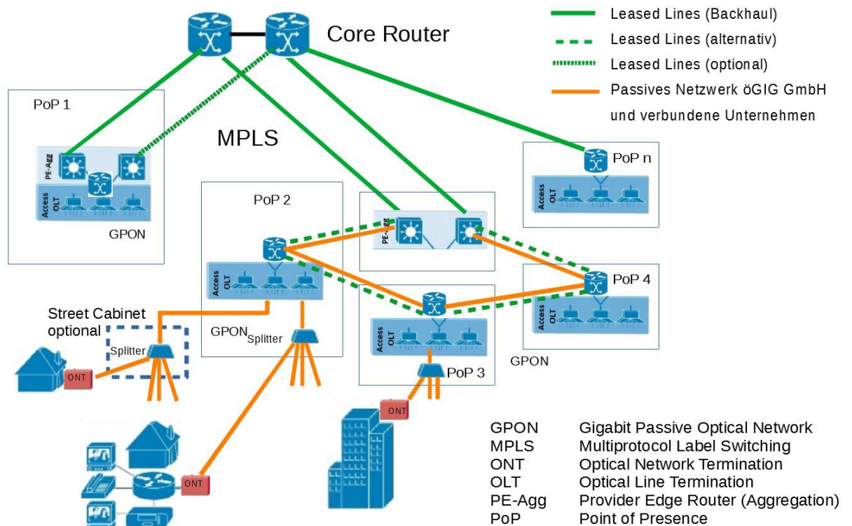
Abbildung 3 beispielhafte Netzwerktopologie
